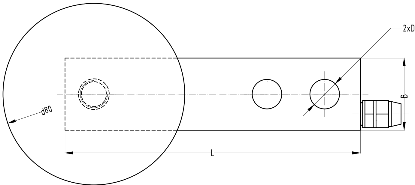
Габаритные характеристики SQС, мм
